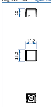
Magneteinheit – Magnet unit
